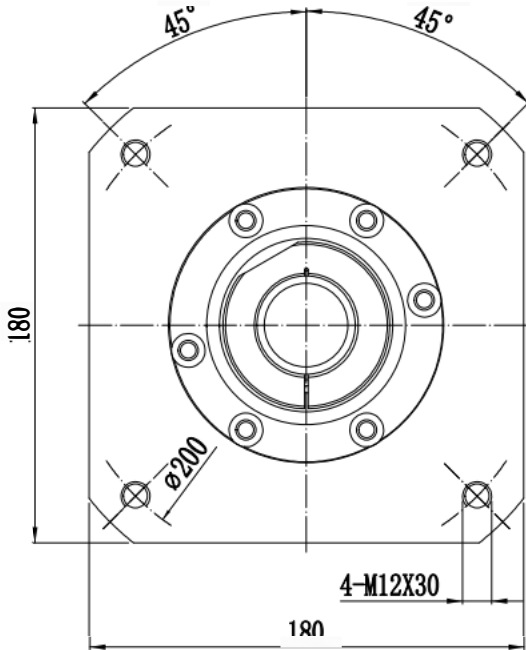
输入端(Input)
